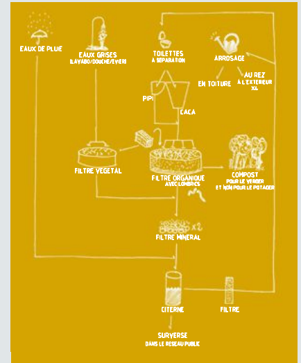
Principe du dispositif d'épuration des eaux. DR
